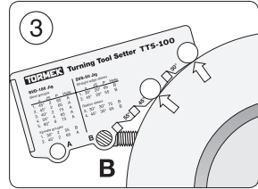
Universalstütze einstellen. Benutzen Sie Loch B.
